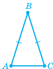
Рис. 168. Рівнобедрений трикутник
